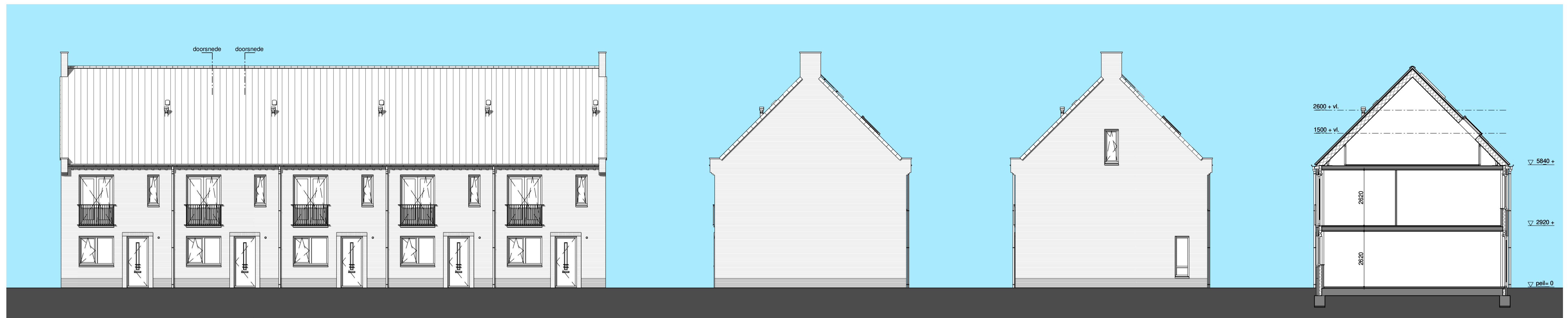
voorgevel - 1:100
