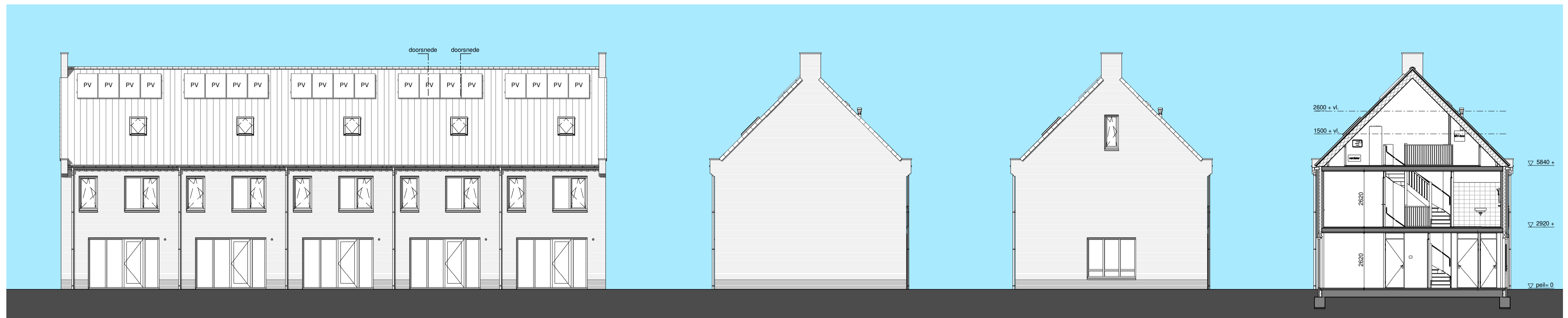
achtergevel - 1:100
