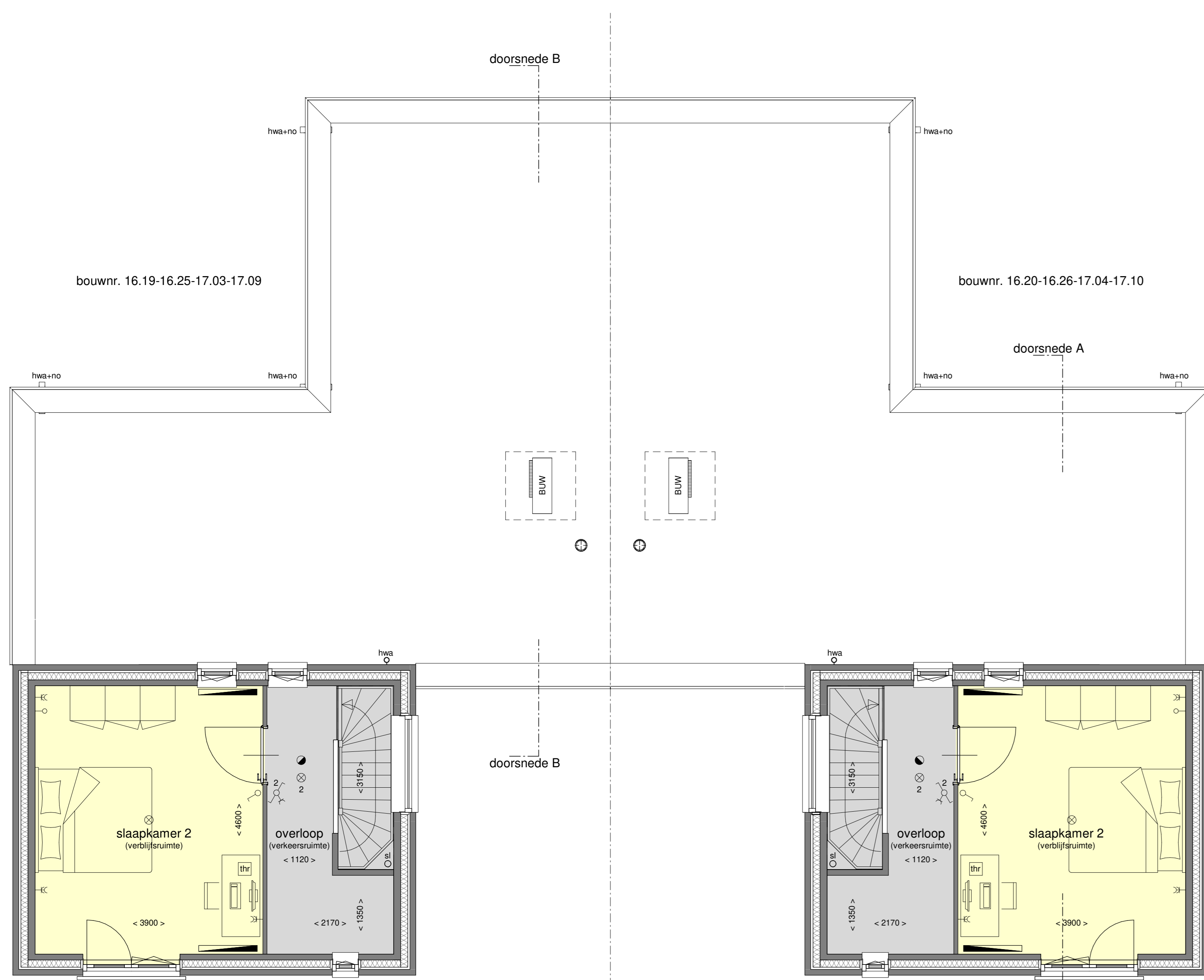
1e verdieping - 1:50 type T
