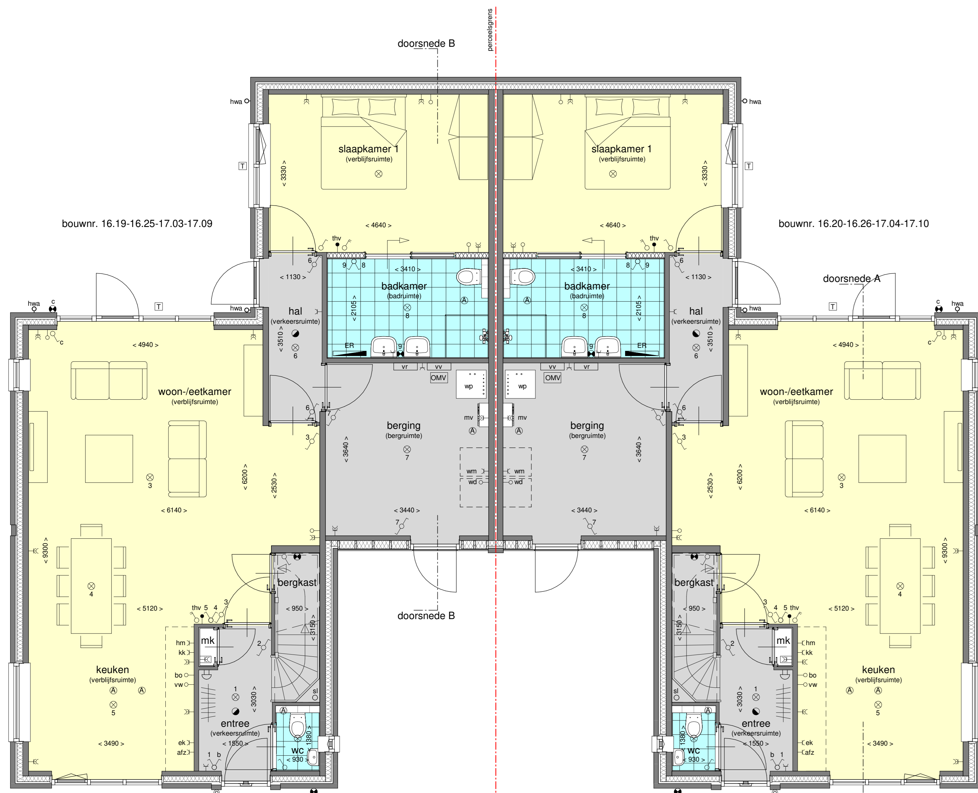
begane grond - 1:50 type T
