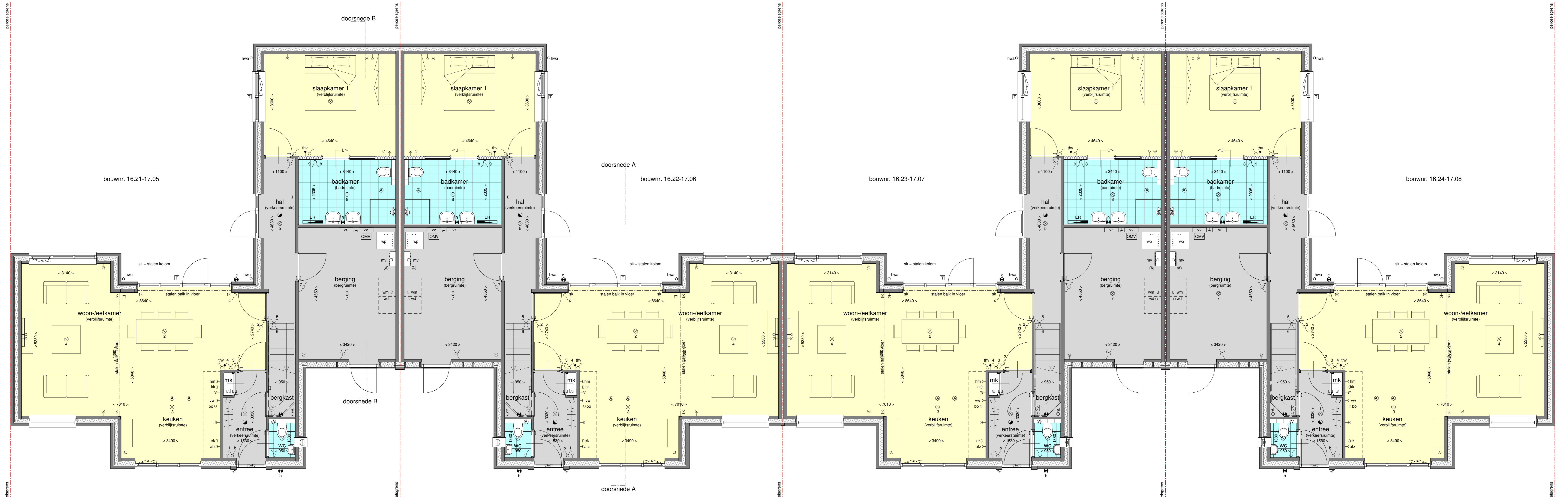
begane grond - 1:50 type V
