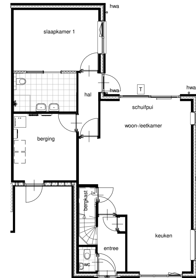
begane grond - woningtype T
