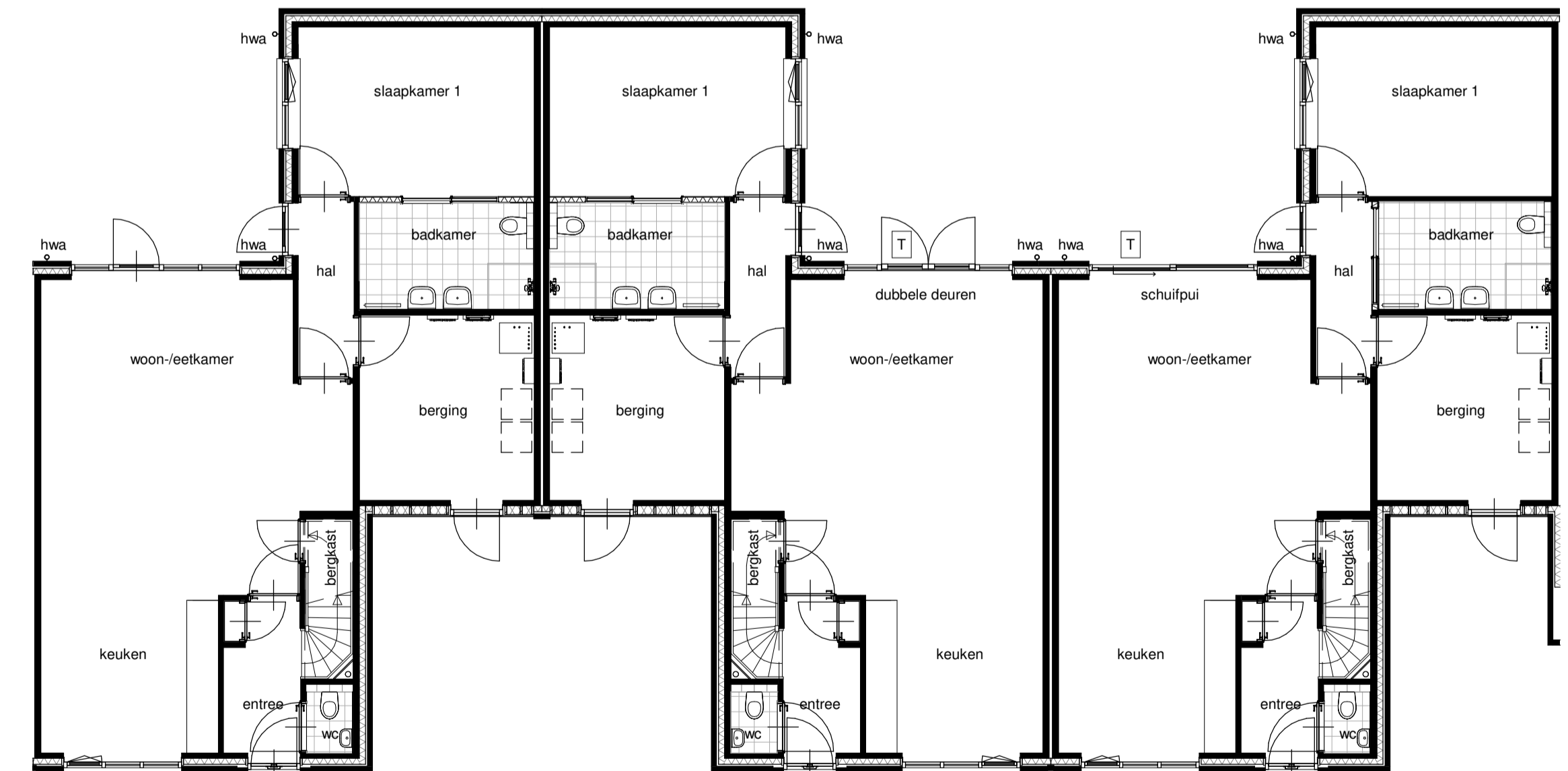
begane grond - woningtype U
