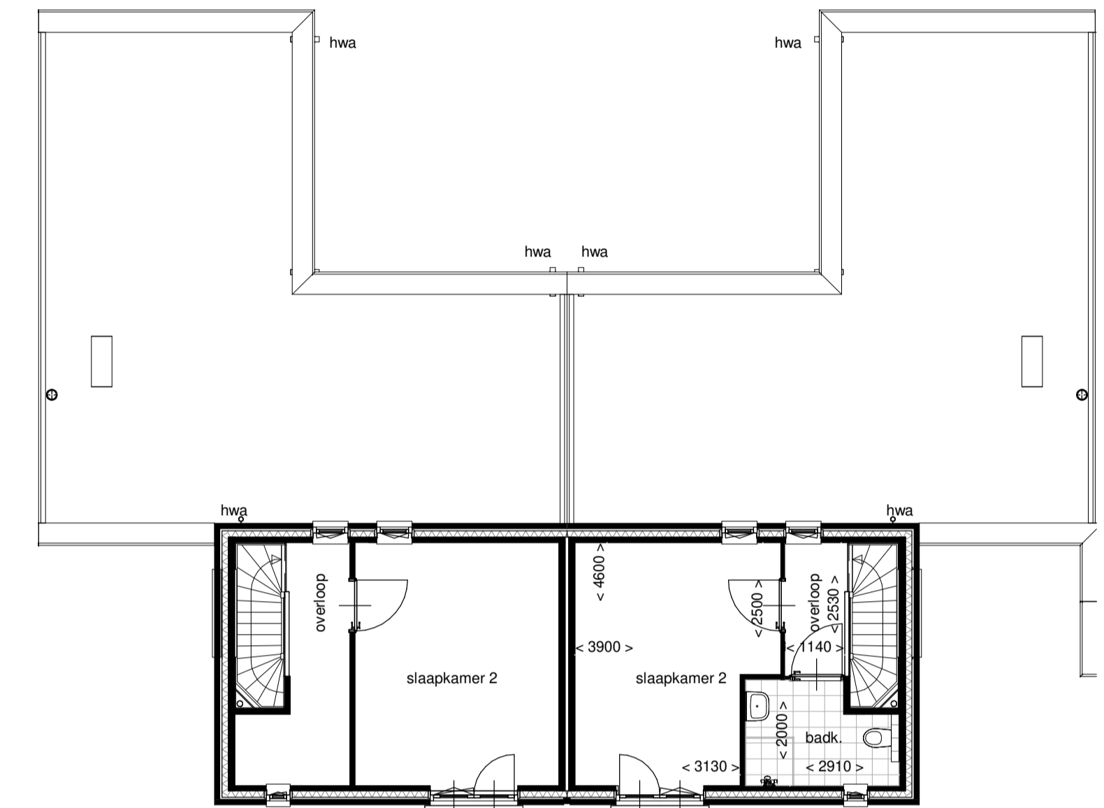
verdieping - woningtype U
