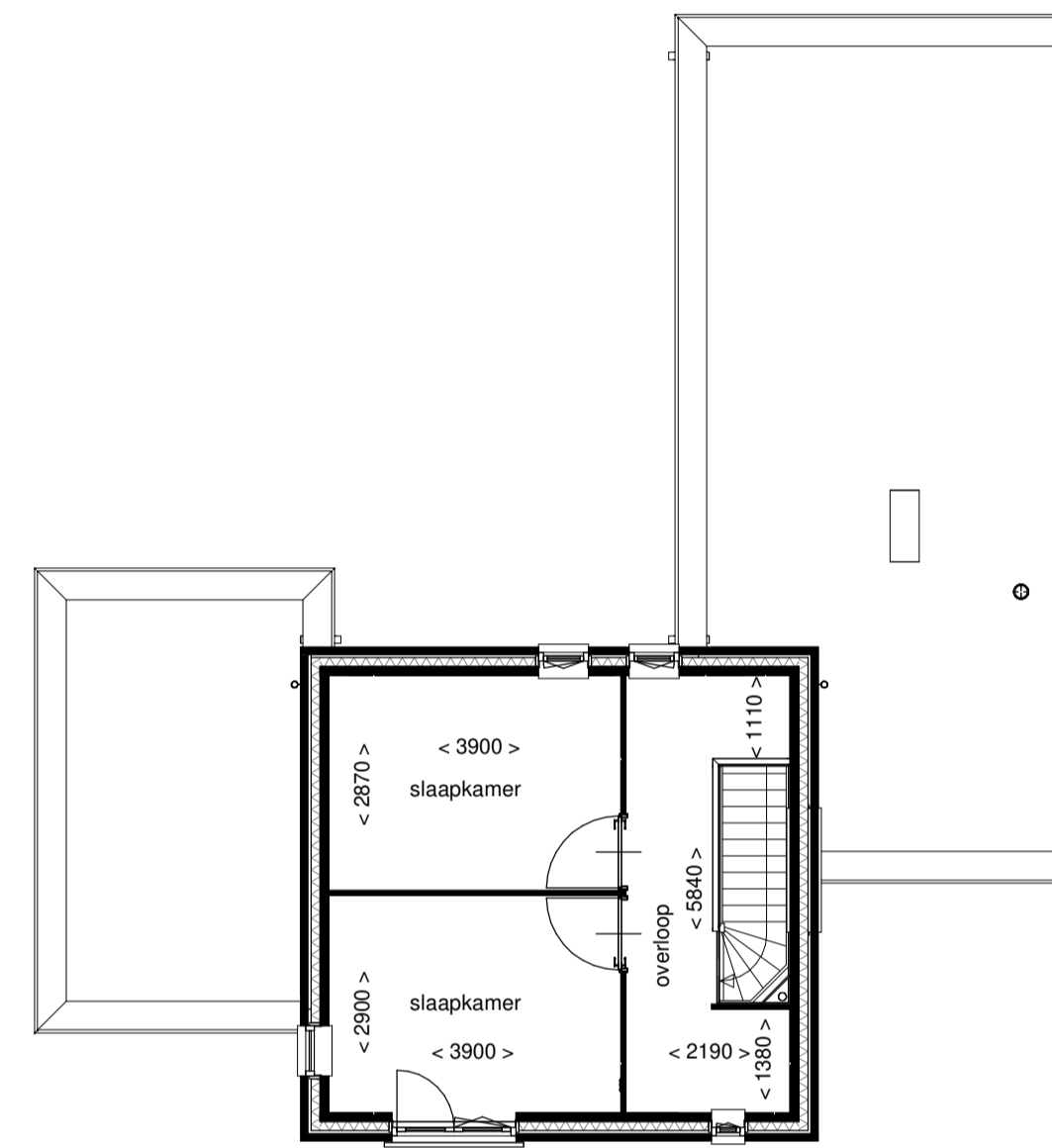
verdieping
