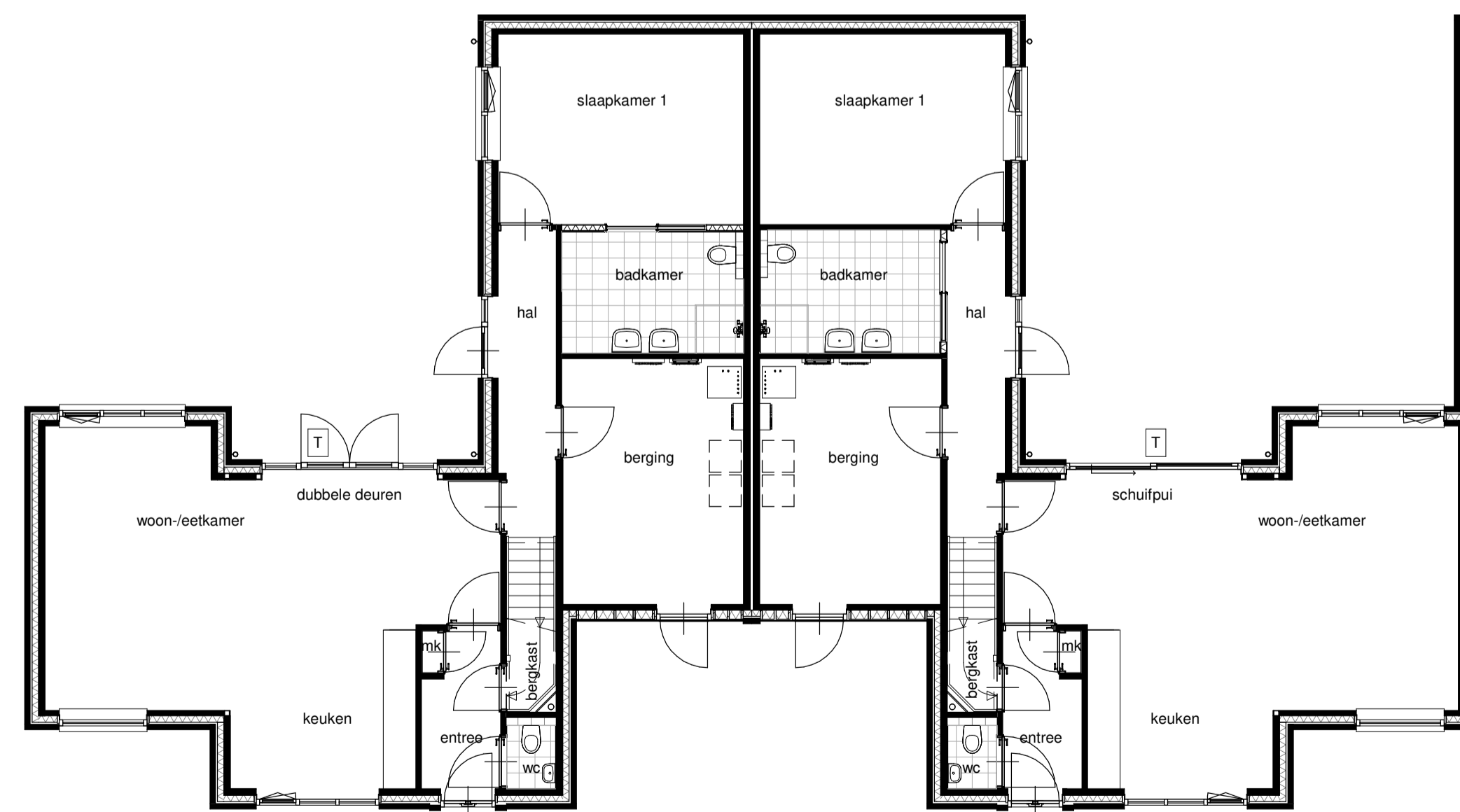
begane grond
