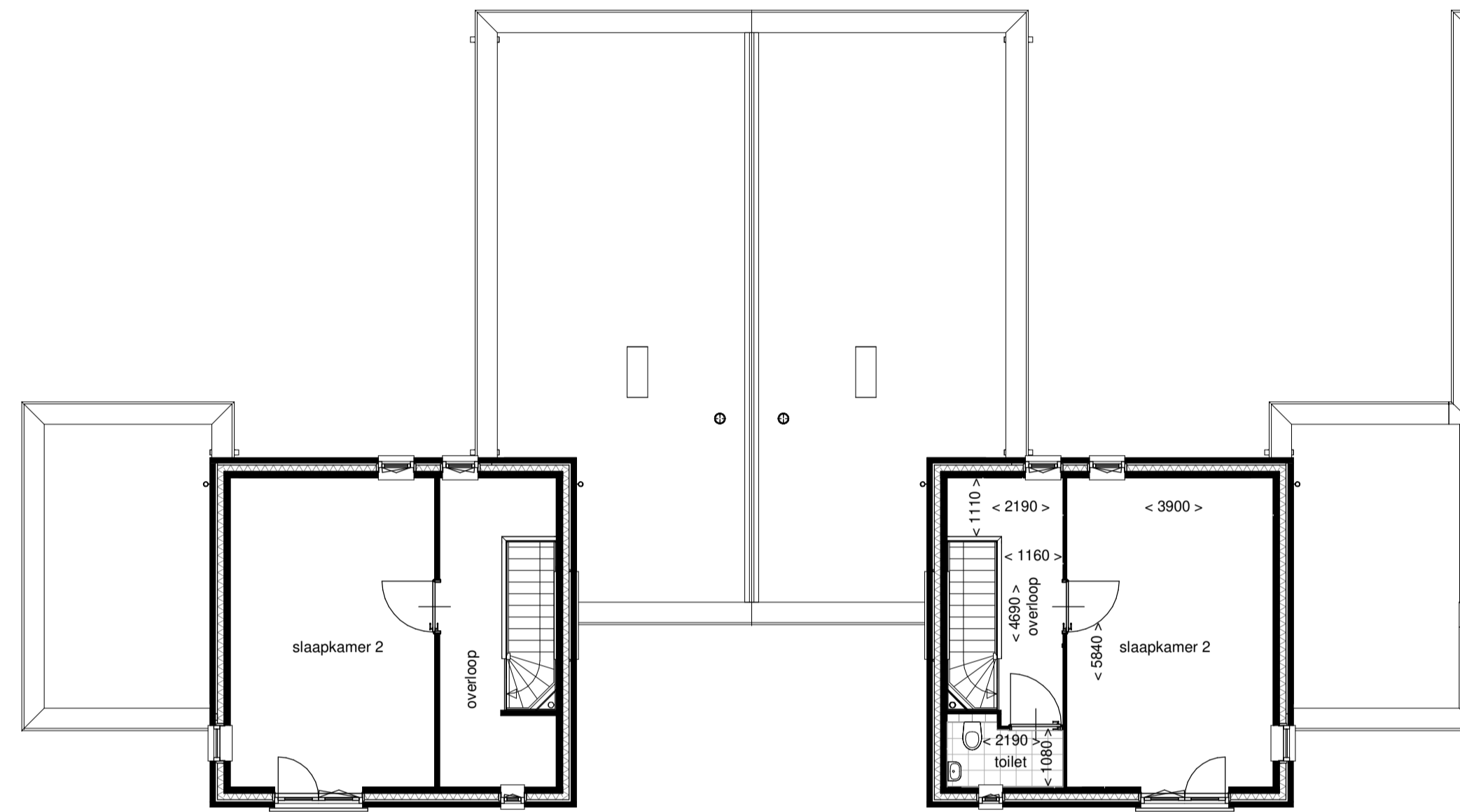
verdieping
