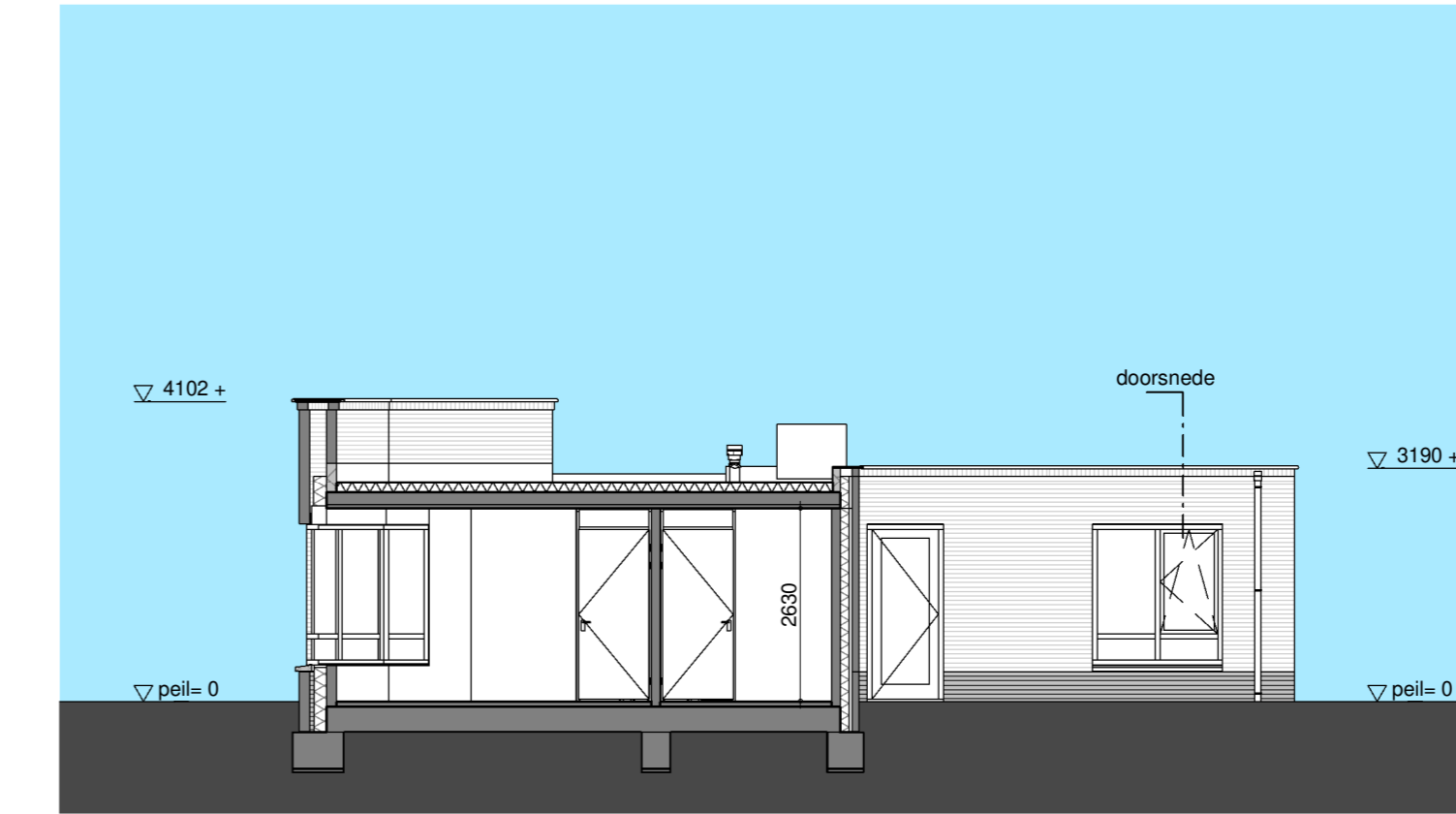
doorsnede / zijgevel - 1:100 bouwnr. 15.03 en 15.09 bouwnr. 15.04 en 15.10 gespiegeld
