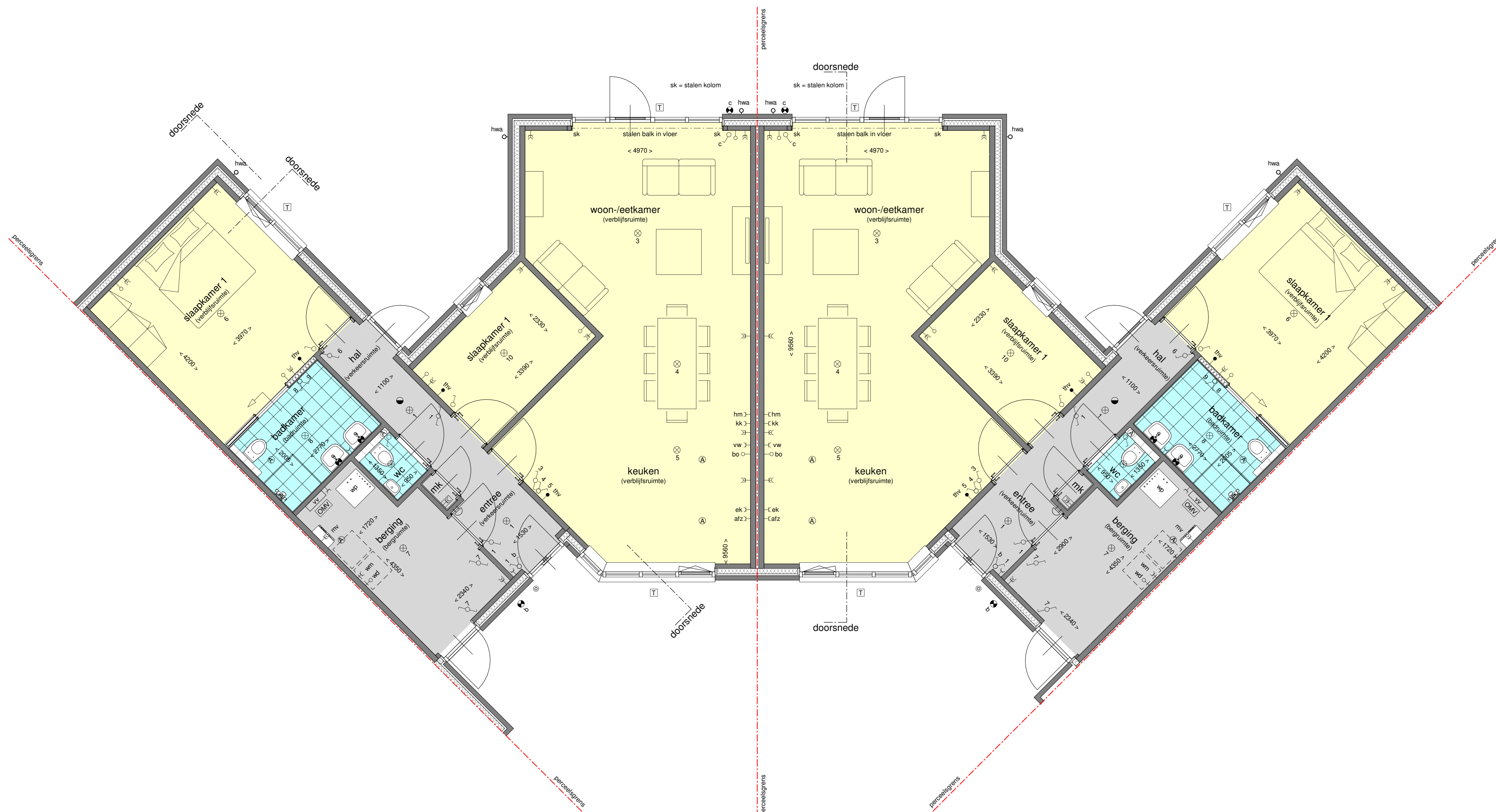
begane grond - 1:50 bouwnr. 15.03 en 15.09
