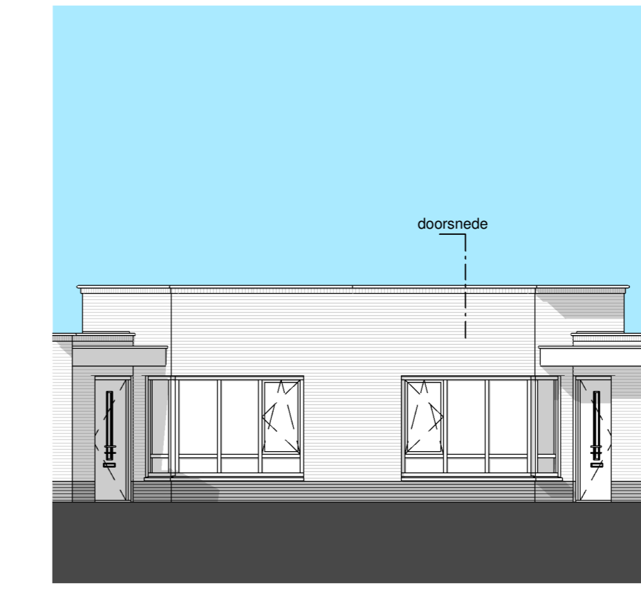
voorgevel - 1:100 bouwnr. 15.03 en 15.09 bouwnr. 15.04 en 15.10
