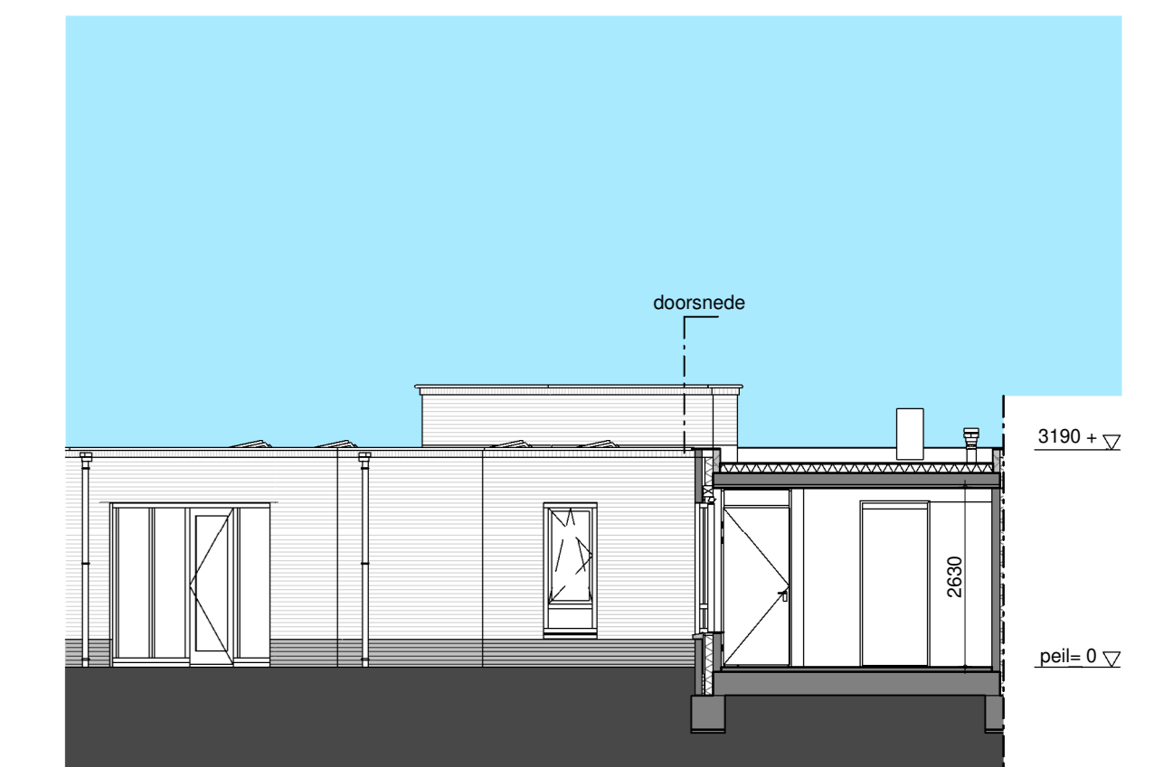
doorsnede / zijgevel - 1:100 bouwnr. 15.03 en 15.09 bouwnr. 15.04 en 15.10 gespiegeld
