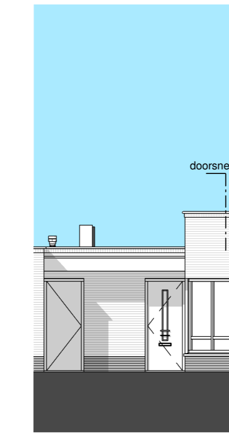
voorgevel - 1:100 bouwnr. 15.03 en 15.09 bouwnr. 15.04 en 15.10 gespiegeld
