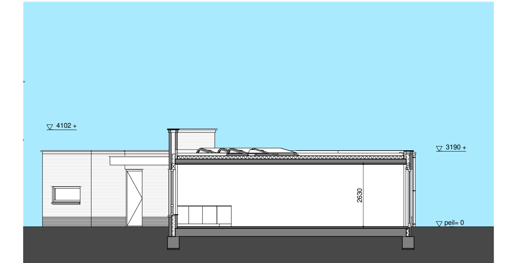
doorsnede / zijgevel - 1:100 bouwnr. 15.04 en 15.10 bouwnr. 15.03 en 15.09 gespiegeld
