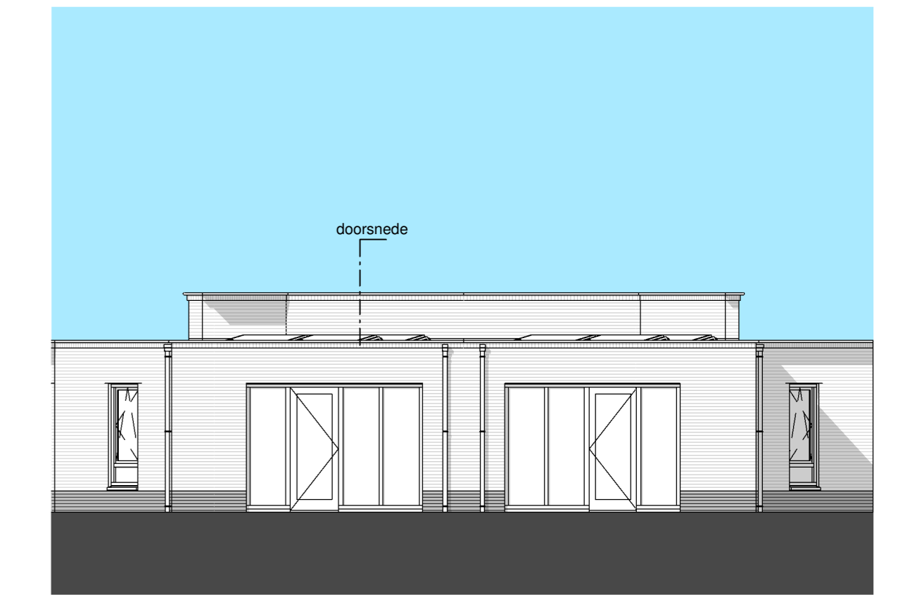
achtergevel - 1:100 bouwnr. 15.04 en 15.10 bouwnr. 15.03 en 15.09
