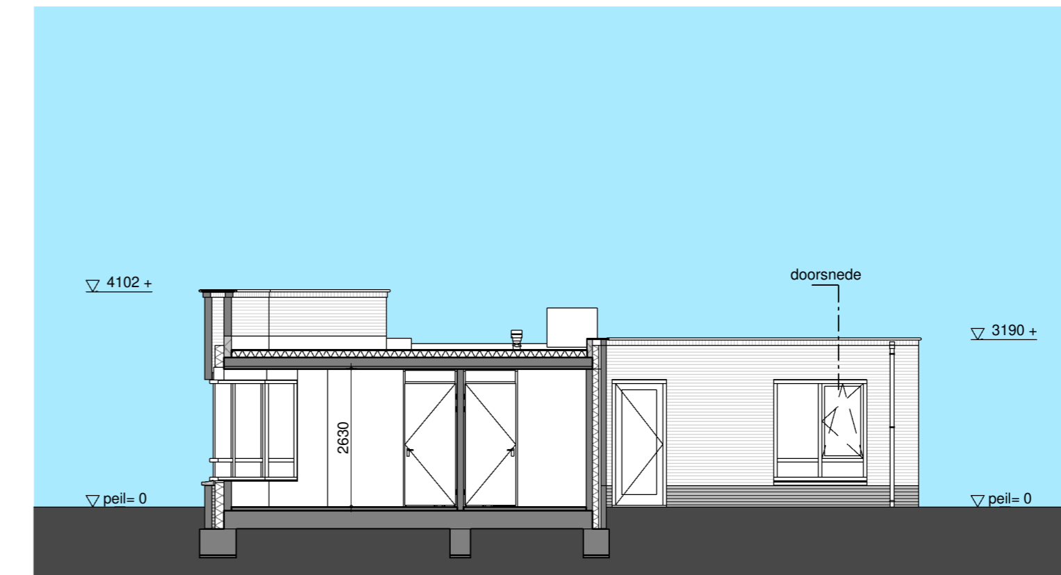
doorsnede / zijgevel - 1:100 bouwnr. 13.17 bouwnr. 13.18 gespiegeld
