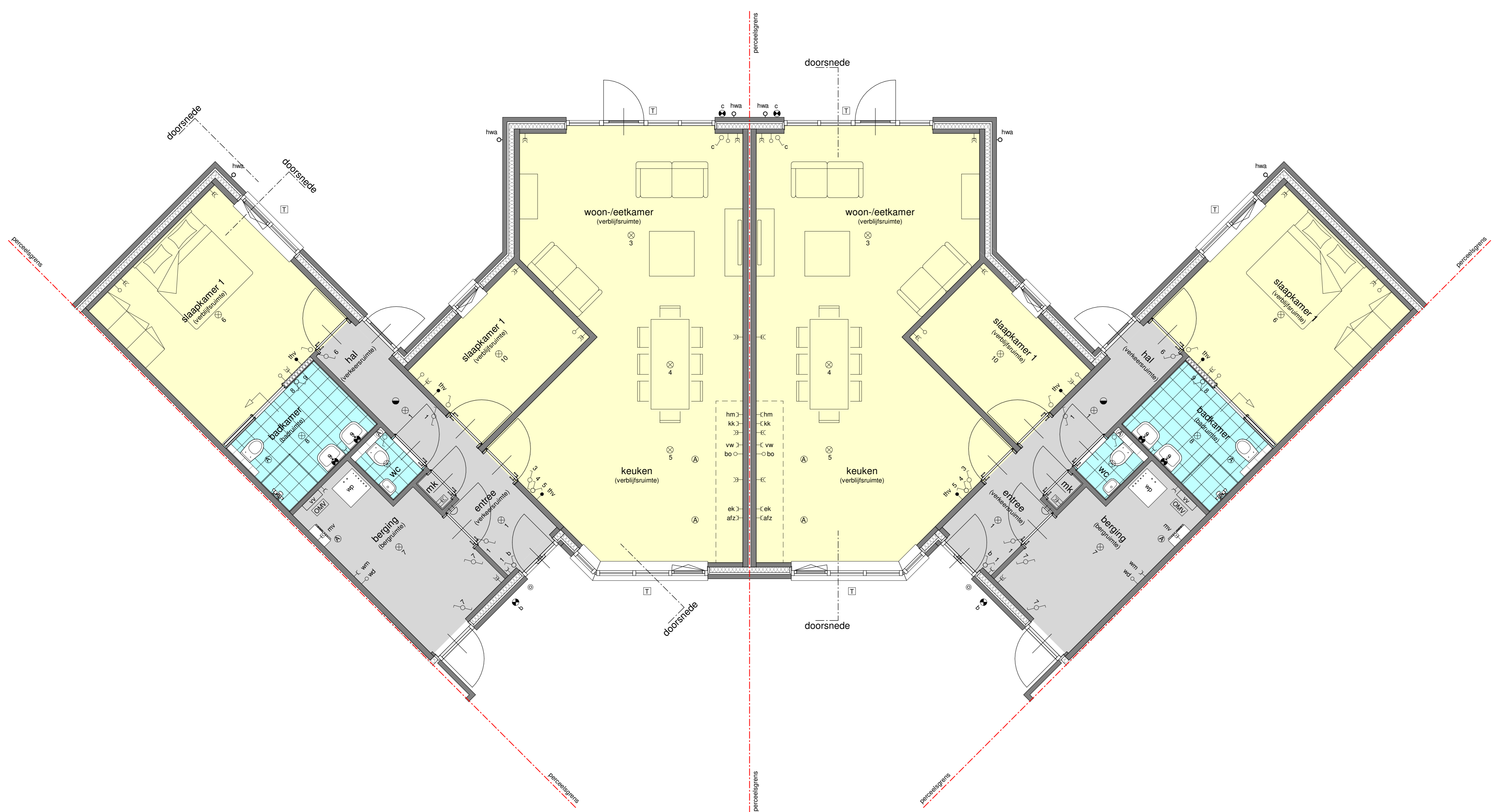
begane grond - 1:50 bouwnr. 13.17
