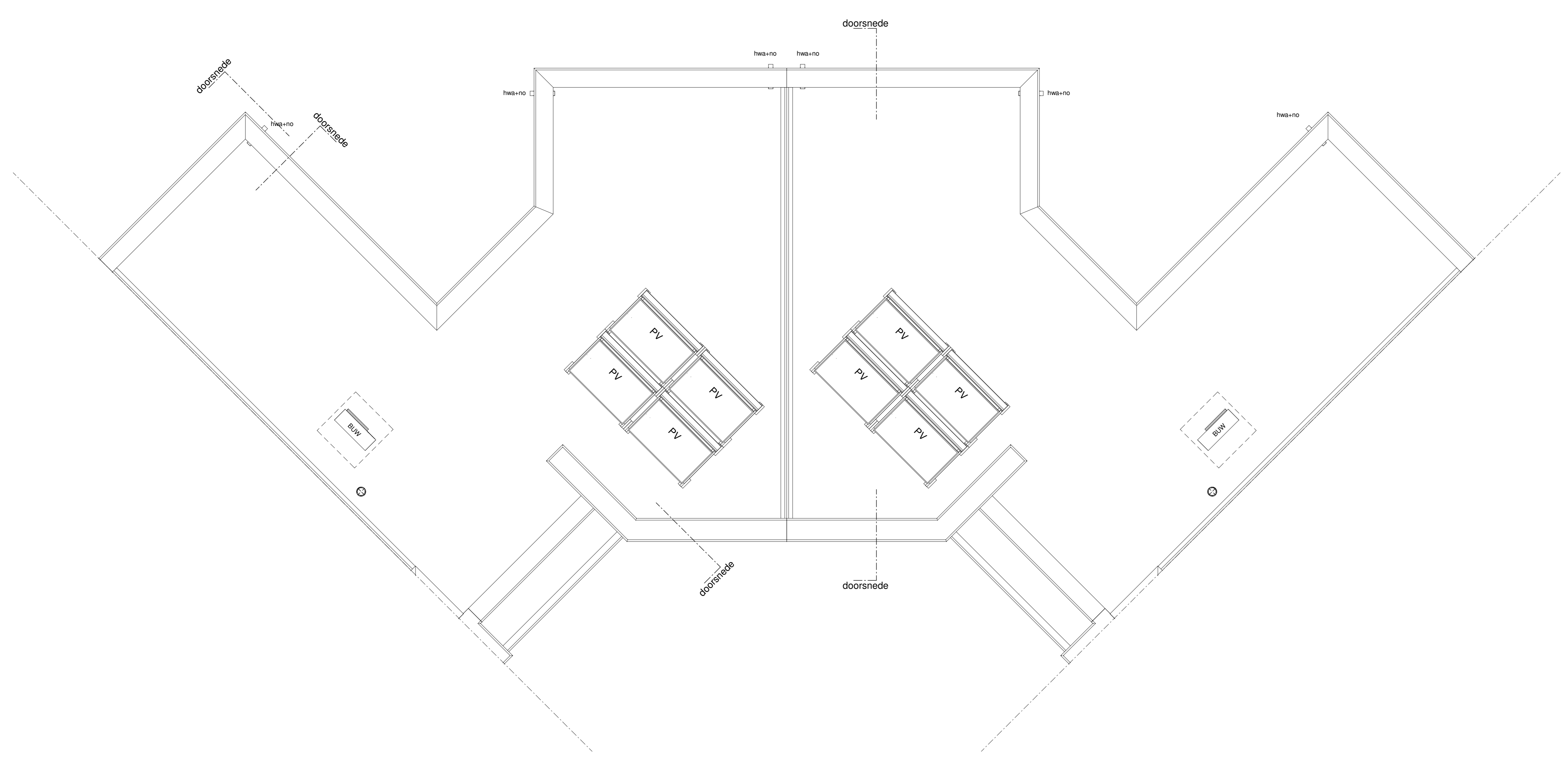
dakaanzicht - 1:50 bouwnr. 13.17
