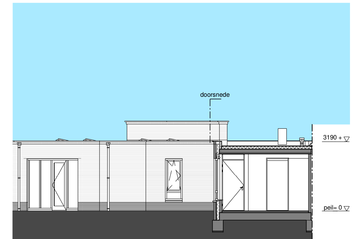
doorsnede / zijgevel - 1:100 bouwnr. 13.17 bouwnr. 13.18 gespiegeld
